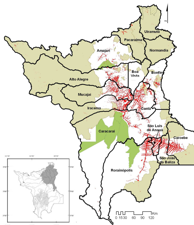
Figura 3. Distribuição espacial do desmatamento entre os municípios de Roraima até 2006. (Base de dados do INPE/Programa PRODES digital). Bege – Terras Indígenas; Verde – Unidades de Conservação Federal; Vermelho – desmatamento; Branco – “áreas de uso” livre. Mapa menor à esquerda representa os grandes tipos de vegetação: Branco – florestas; Cinza escuro – savanas; Cinza claro – campinas e campinaramas (Fonte: BARBOSA et al. , 2008).
